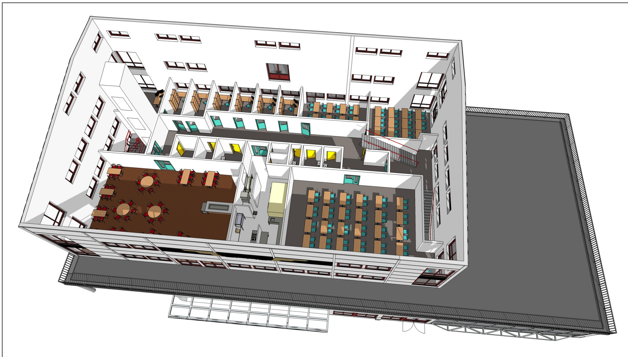
2. etasje
